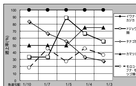
図5 双翼型隔壁における魚種別遡上率
