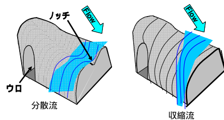
図8 双翼型魚道のノッチ効果
