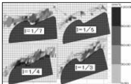
図6 勾配と流況(ベクトル・コンター)
