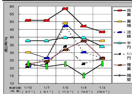
図4 隔壁形状と遡上率
