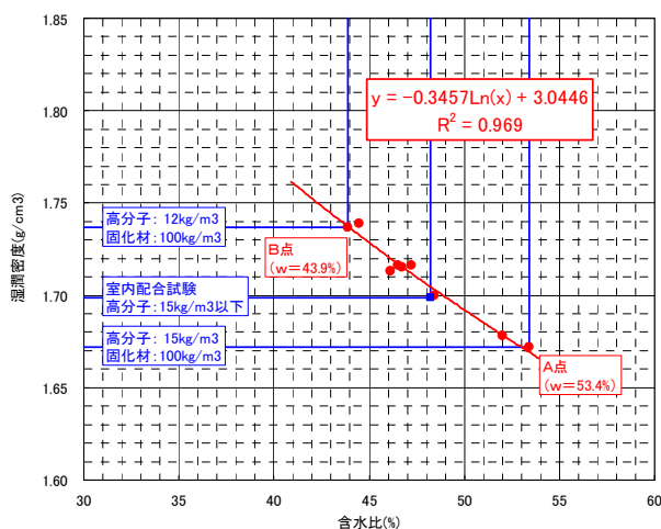
図-1 排泥の湿潤密度と含水比の関係（工事着手時）
