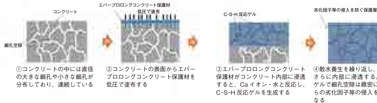
(図-1) EP保護材のコンクリート内部での浸透・改質メカニズム
