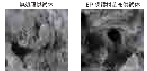
(写真-3) 走査型電子顕微鏡写真 (SEM像：倍率15000倍)
